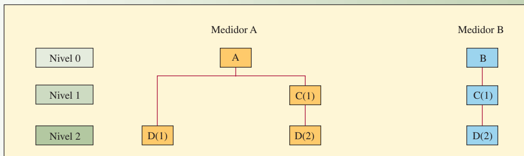
La ilustración muestra los subensamblés y las piezas que componen los medidores y se indica entre paréntesis el número de unidades necesarias por unidad antecesora.
